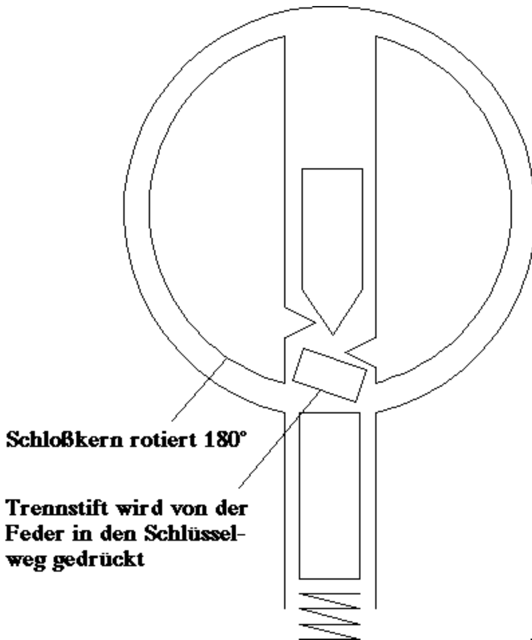
Bild 9.9: Der Trennstift- oder Gehäusestift kann in den Schlüsselweg eintreten
