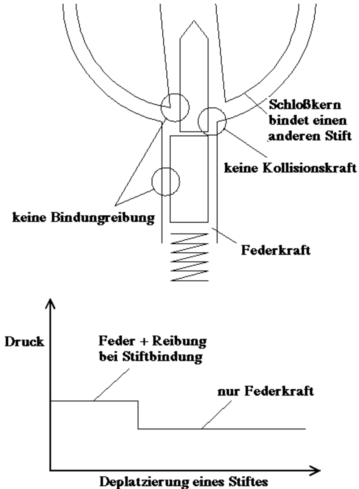
Bild 9.3: Der Gehäusestift ist breiter als der Kernstift
