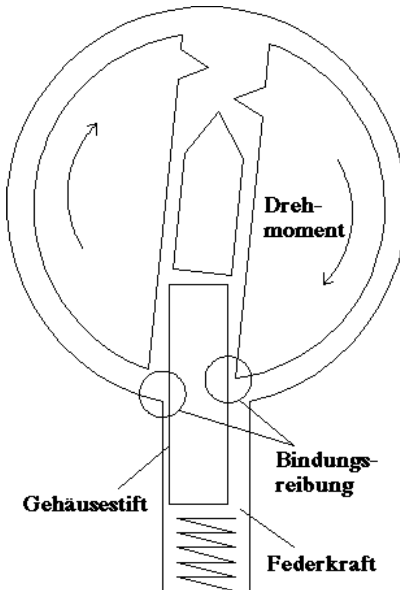
Bild 5.2: Der Gehäusestift ist eingeklemmt
