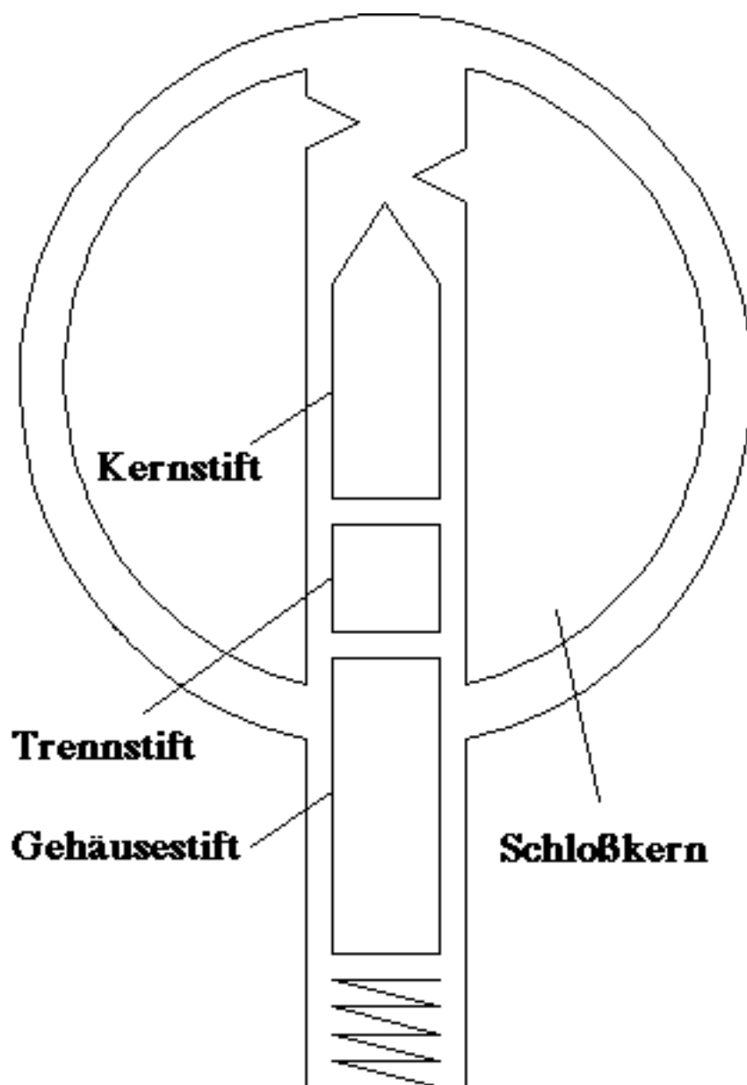
Bild 9.8: Trennstiftstifte für Generalschlüssel
