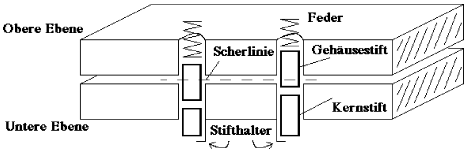
Bild 3.1 : Ebenenmodell eines Schlosses
