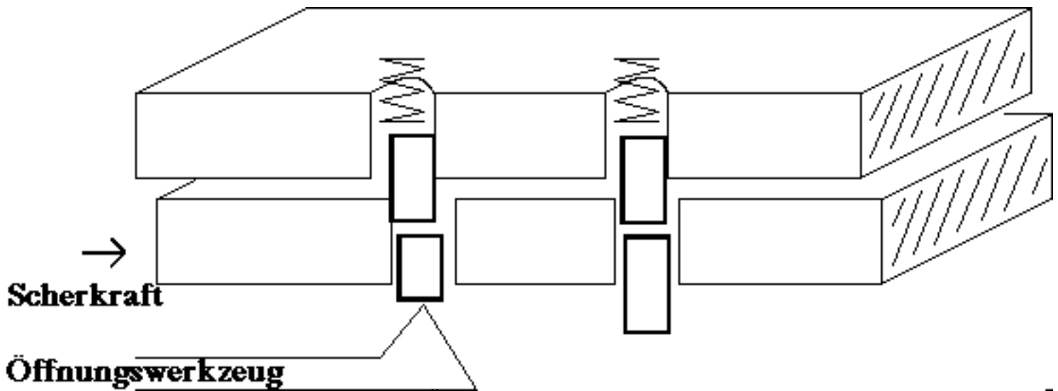
Bild 4,2: (b) Das Öffnungswerkzeug hebt den Kernstift
