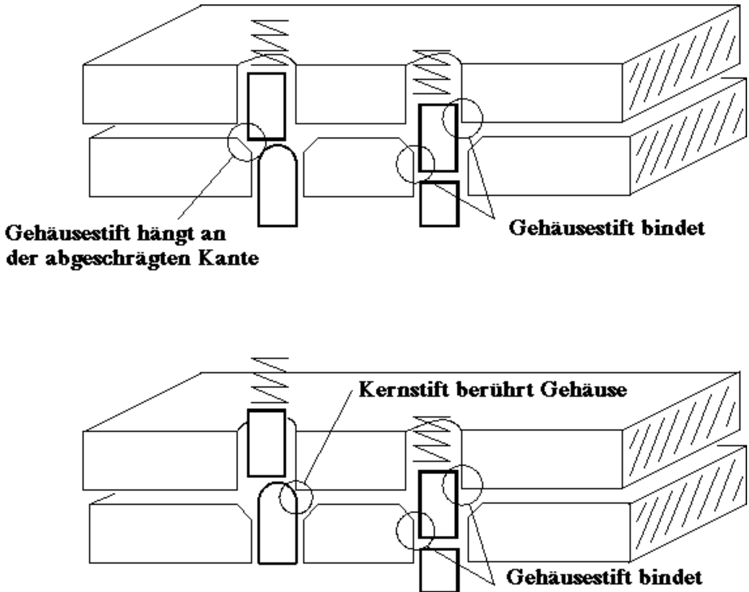
Bild 9.4: Abgeschrägte Schlosskernlöcher und abgerundete Kernstifte
