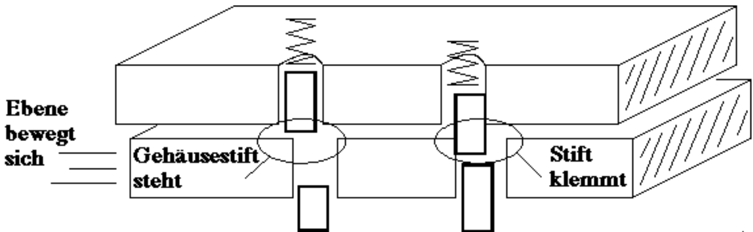
Bild 4,3: (c) Linker Gehäusestift sitzt, der rechte ist richtig eingeklemmt
