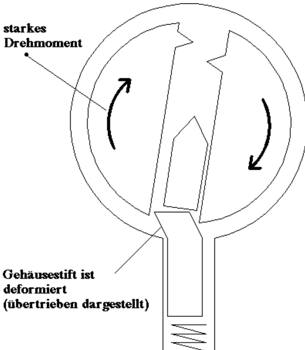
Bild 9.2: Der Gehäusestift ist durch elastische Deformation falsch gesetzt
