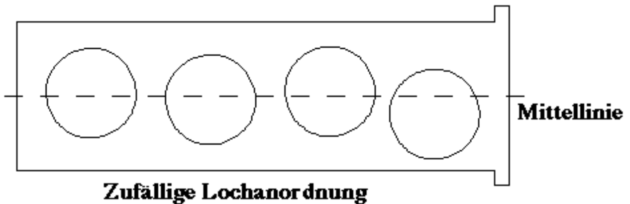
Bild 6.2: Ausrichtung der Löcher im Schlosskern
