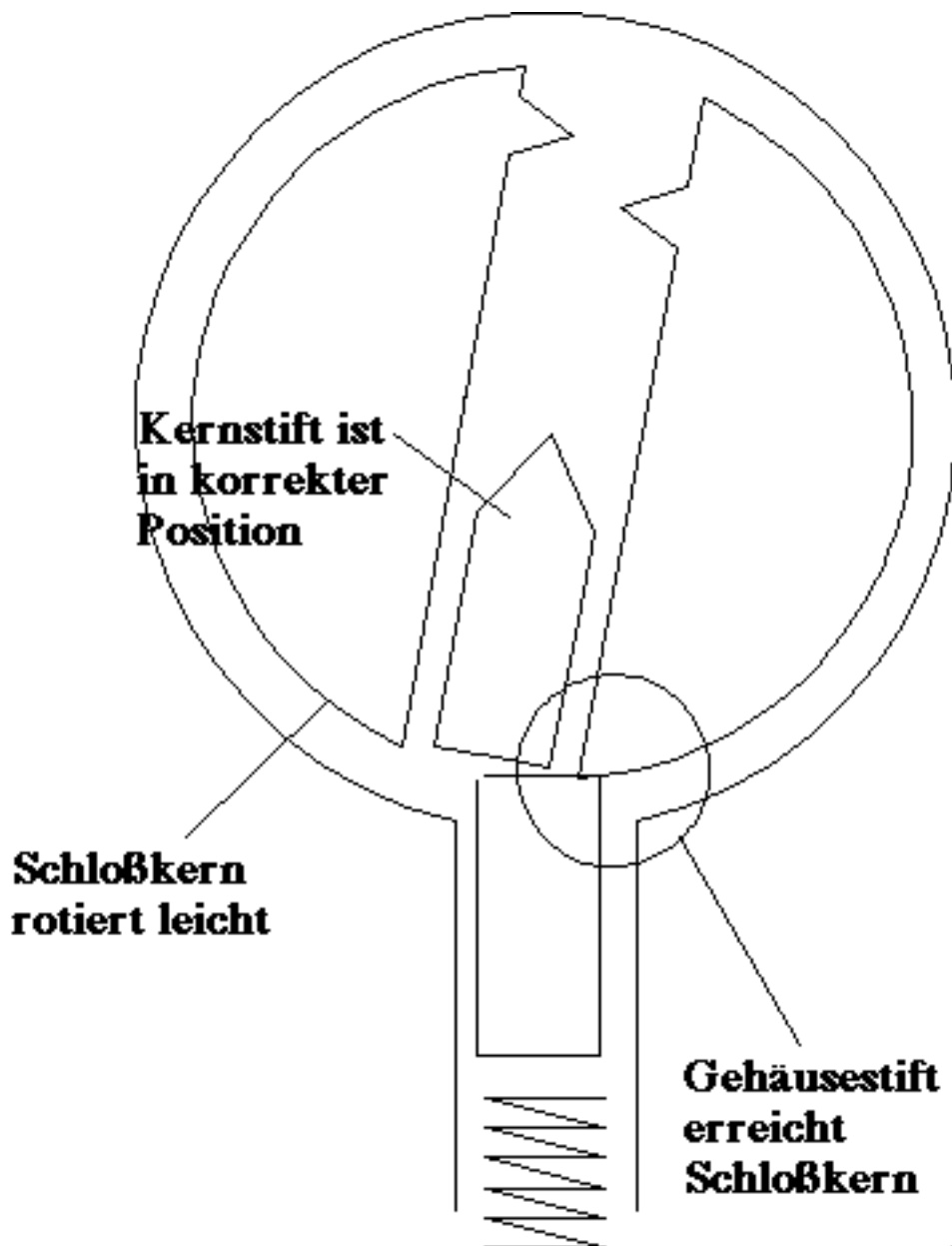
Bild 6.1: Der Kernstift befindet sich im Schlosskern
