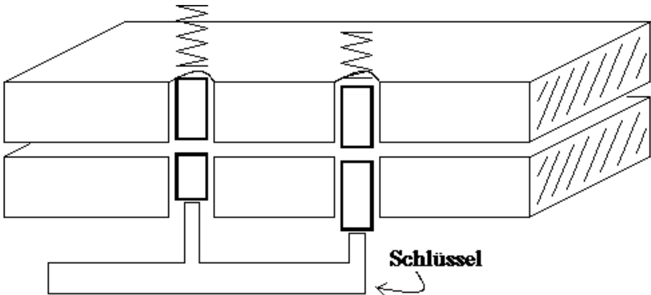
Bild 3.2 : (a) Der Ebenenschlüssel hebt den Stift
