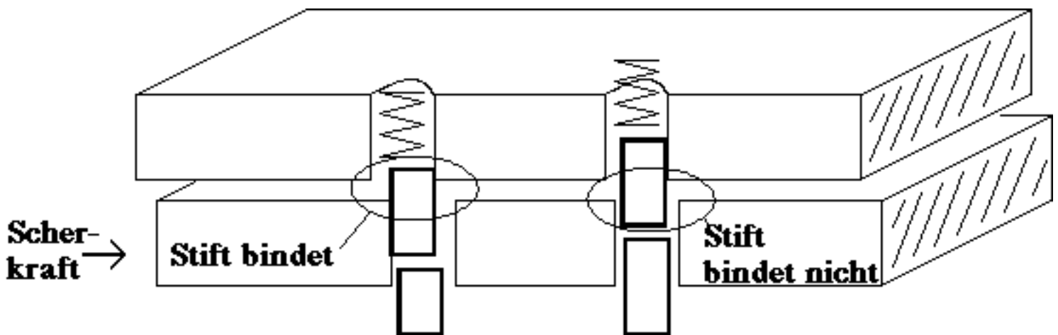
Bild 4,1: (a) Einfache Kraft, die den Gehäusestift bindet
