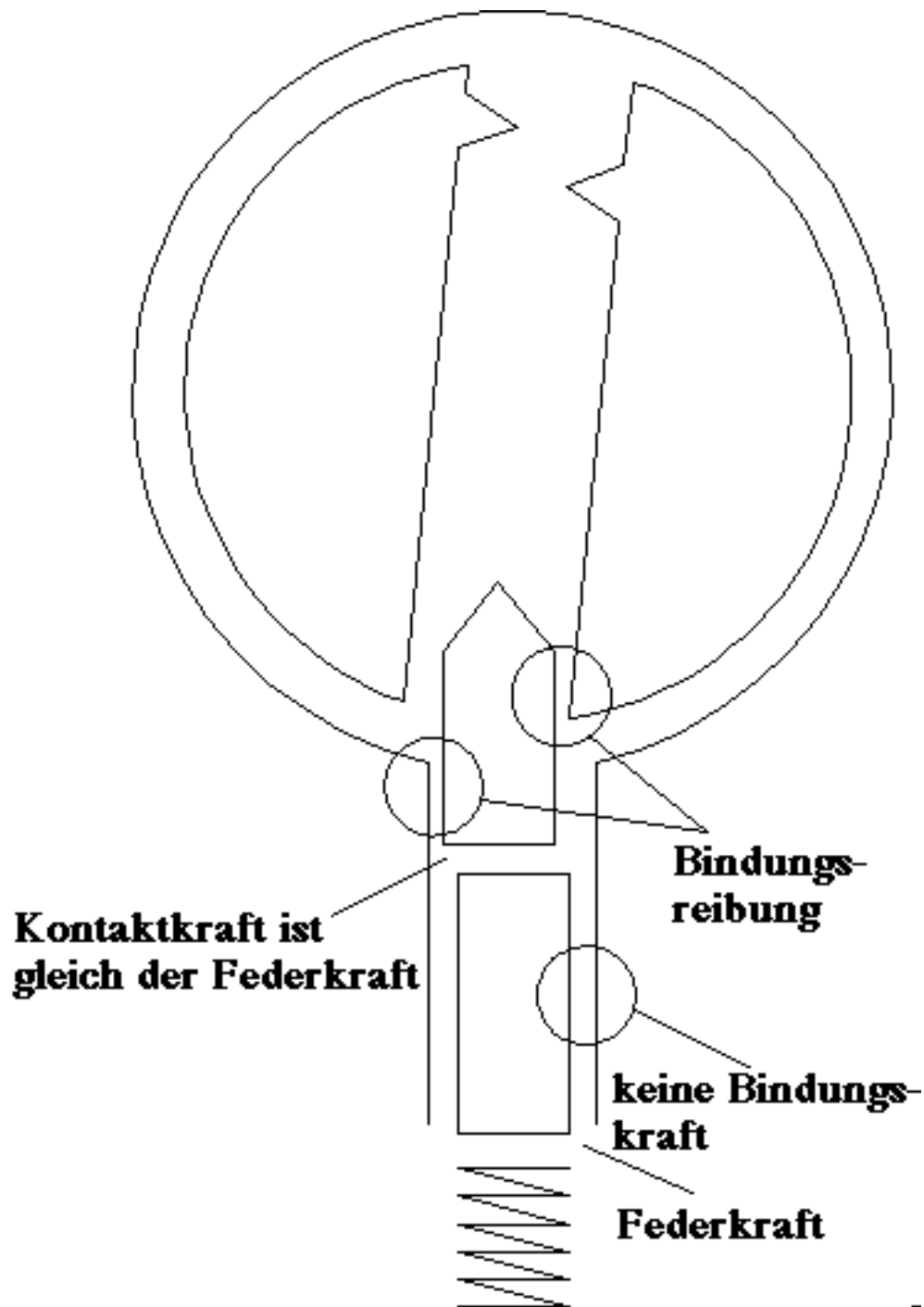
Bild 5.4: Kernstift tritt in das Schlossgehäuse ein
