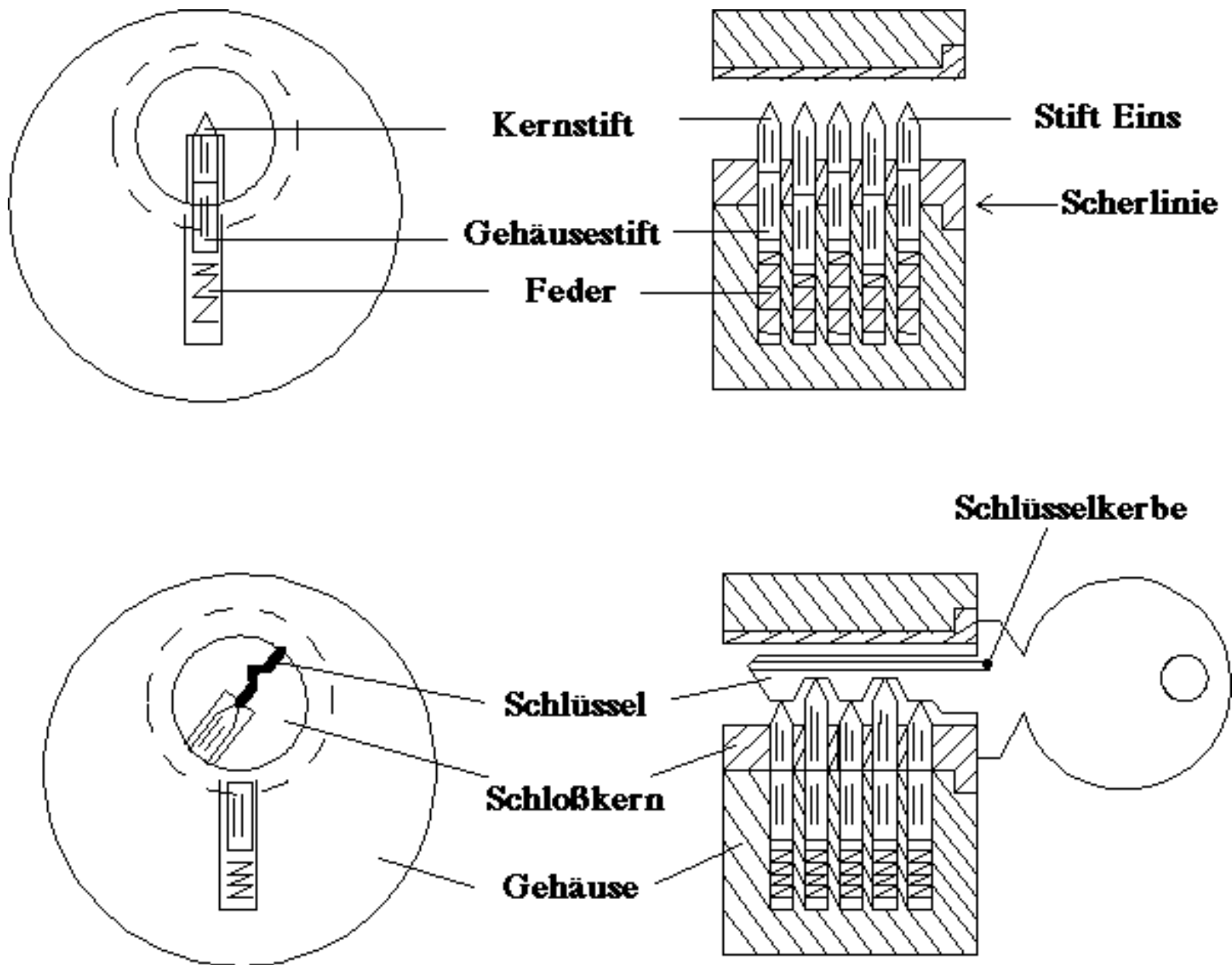
Bild 2.1: Arbeitsweisen von Stiftzuhaltungsschlössern
