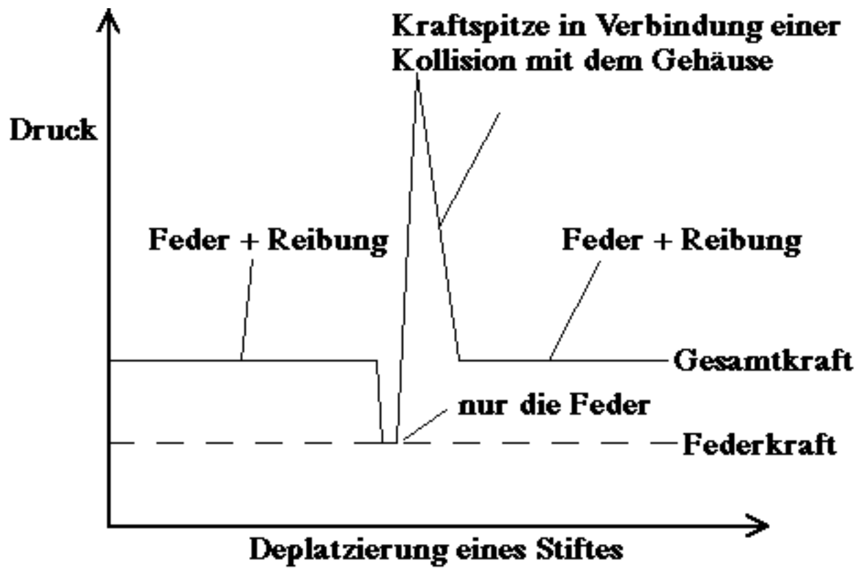
Bild 5.5: erforderlicher Druck, die Stifte zu bewegen
