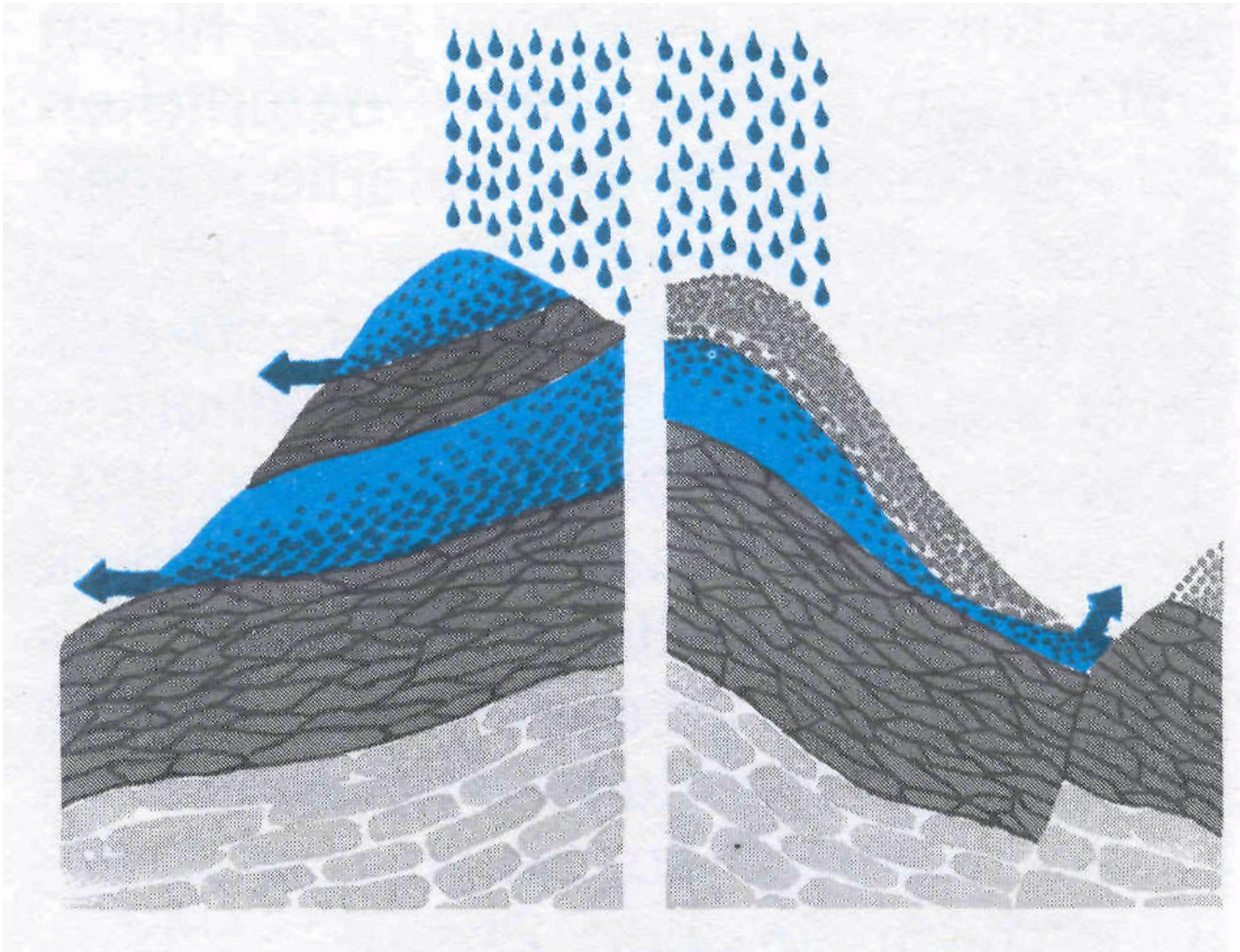
Quellen entspringen, wo wasserführende Schichten direkt austreten (links) oder nach einem Faltenbruch (rechts) an die Erdoberfläche dringen.
