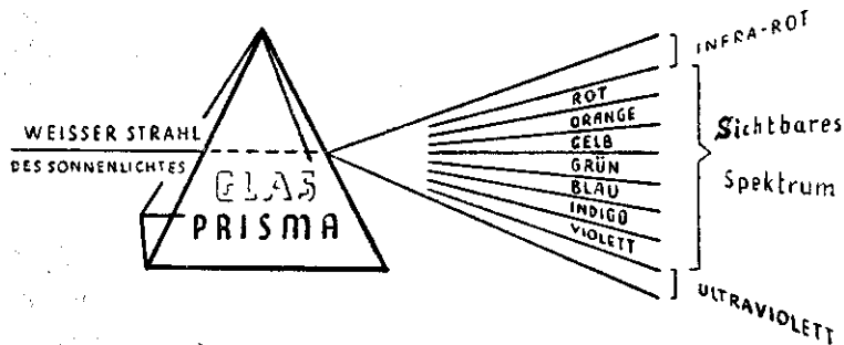
Abb. 53. Die Spektralfarben des Sonnenlichtes.
