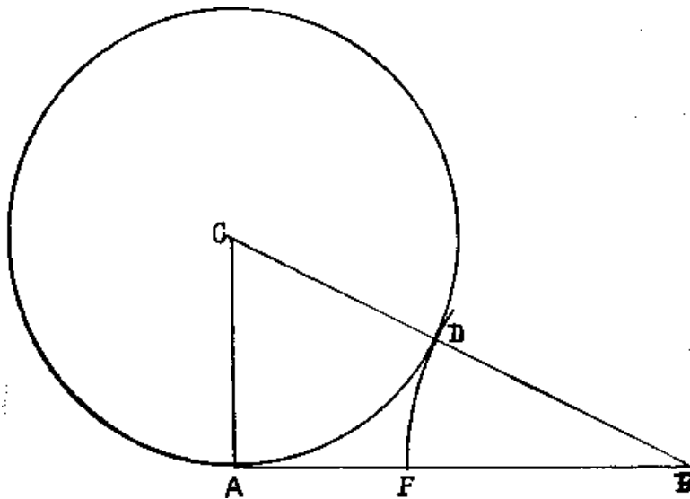
Abb.3a. Der Goldene Schnitt.
