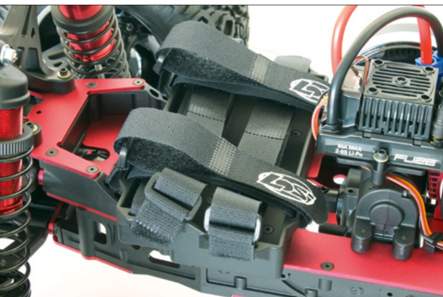
Vier Klettbänder halten die LiPos sicher in der großzügigen Akkubox
