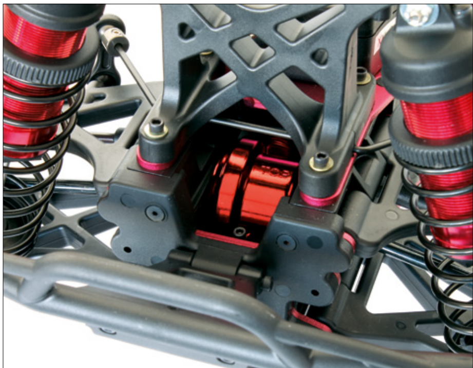
In magentafarbenen Alugehäusen vorne und hinten sitzt jeweils ein Kegelraddifferenzial
