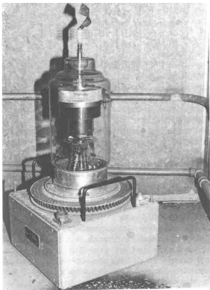
Thyratron
