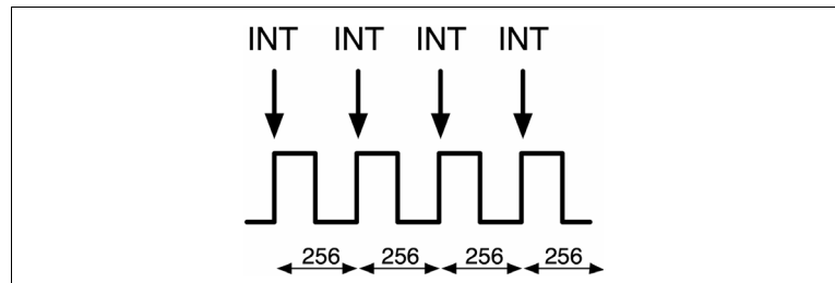
Abbildung 10-4 ► Aufruf der Interrupt-Routine
