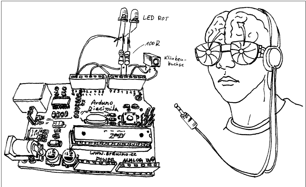
▲ Abbildung 4-5 Brainmachine Schaltung
