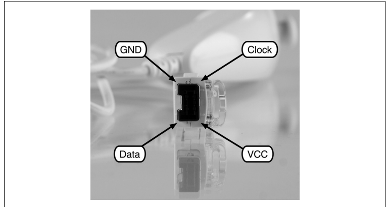
Abbildung 9-7 ► Nunchuck-Pinbelegung
