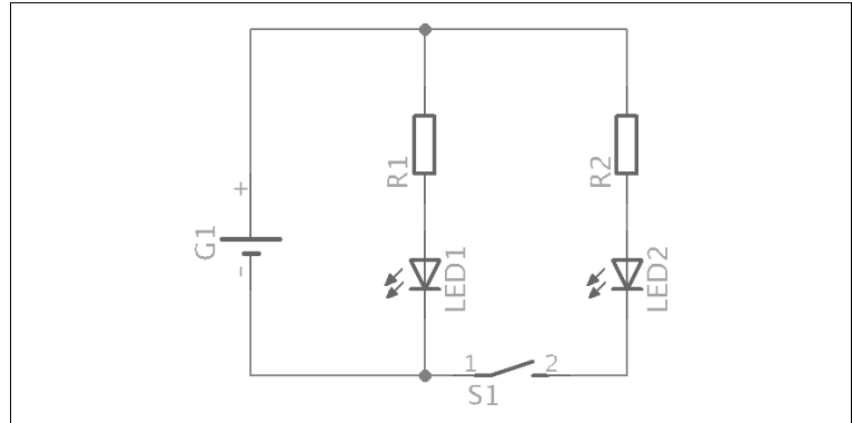
Abbildung 2-5 ► LED-Schaltbild
