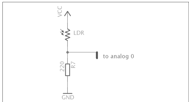
Abbildung 5-6 ► Lichtsensor-Aufbau
