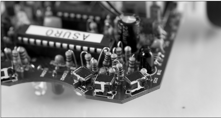
◀ Abbildung 8-5 Asuro-Taster
