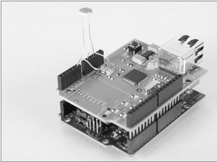
◀ Abbildung 6-3 Twitterserver-Aufbau
