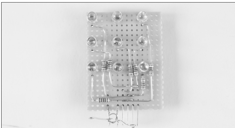
◀ Abbildung 7-2 Würfelaufbau, Lochrasterplatine oben
