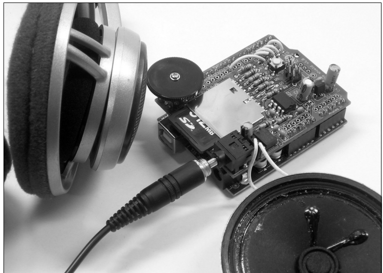
Abbildung 9-2 ► Arduino WaveShield
