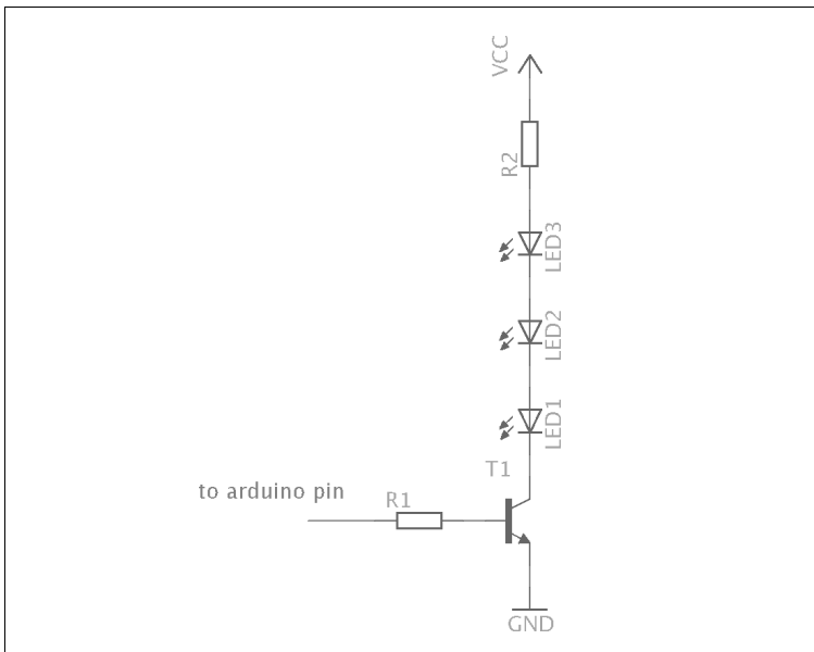
◀ Abbildung 3-7 Transistorausgangsschaltung
