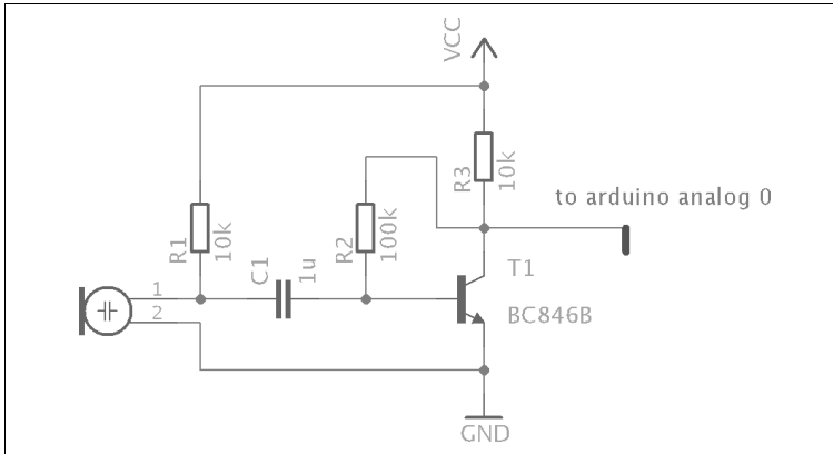
◀ Abbildung 4-3 Tamagotchi-Schaltung
