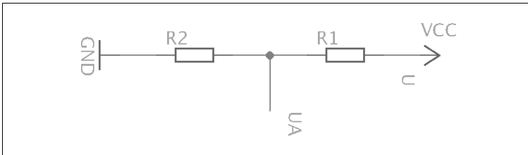
◀ Abbildung 2-4 Spannungsteiler
