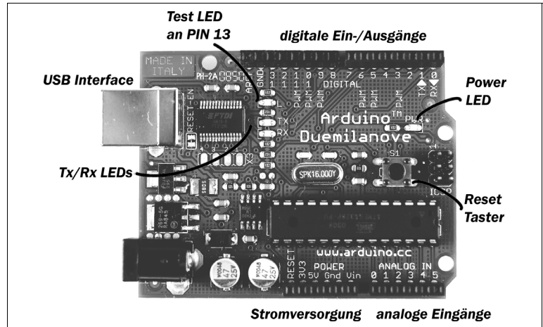
Abbildung 1-3 ► Das Arduino-Board mit seinen einzelnen Bestandteilen
