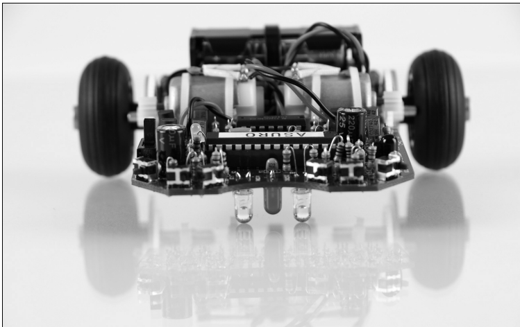
◀ Abbildung 8-1 Asurino
