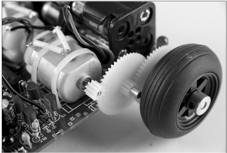
Abbildung 8-4 ► Asuro-Zahnräder
