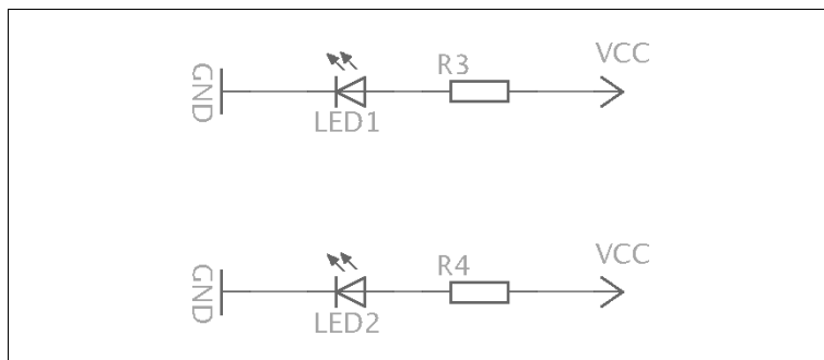
◀ Abbildung 2-6 Schaltbild mit Spannungs- versorgungssymbolen
