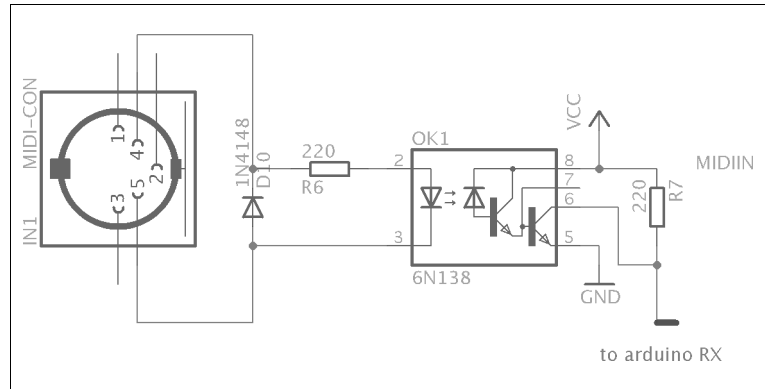
Abbildung 9-4 ► Schaltbild MIDI-Input
