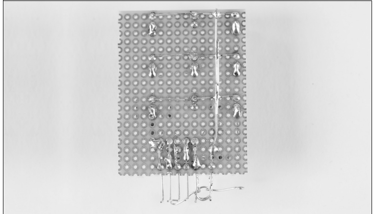
Abbildung 7-3 ► Würfelaufbau, Lochrasterplatine unten
