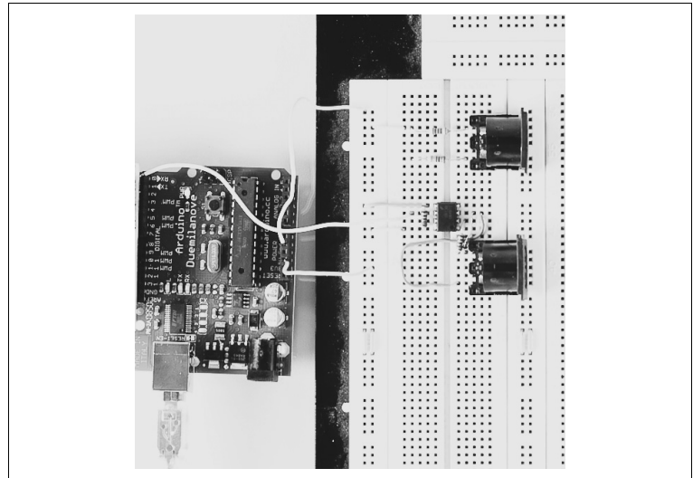
Abbildung 9-5 ► Schaltung MIDI-Input und MIDI-Output
