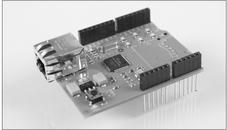
Abbildung 6-1 ► Ethernet-Shield
