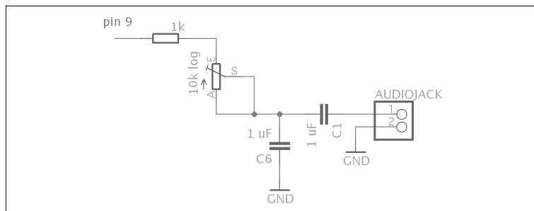
Abbildung 10-1 ► Schaltplan (ohne Steuerung)
