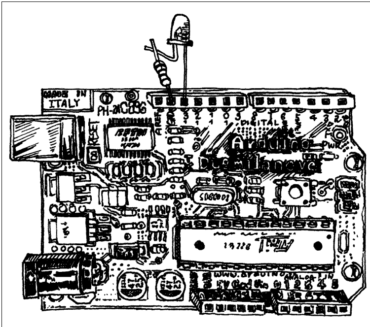
◀ Abbildung 3-1 Arduino-Board
