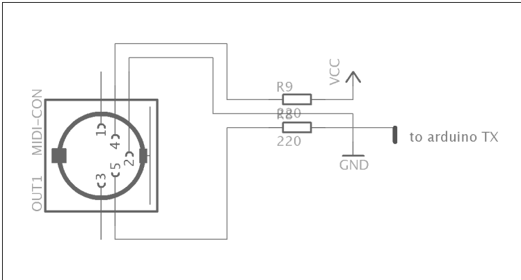
◀ Abbildung 9-6 Schaltbild MIDI-Output
