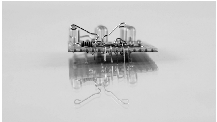
Abbildung 7-4 ► Rüttelsensor
