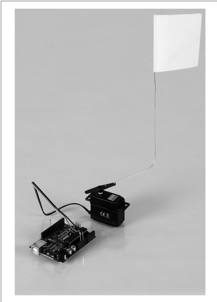
◀ Abbildung 5-4 Gobetwino-Aufbau
