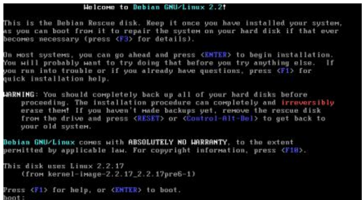
Abbildung 2-6. Bootmenü
