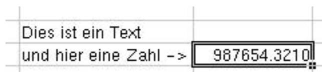
Abbildung 11-1. Gnumeric Eingabe
