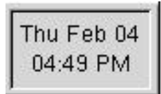
Abbildung 6-10. Uhr-Applet
