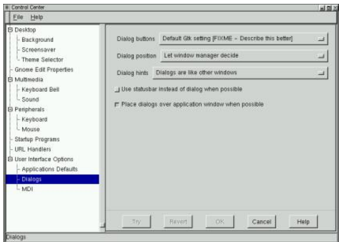
Abbildung 6-38. Capplet Dialog
