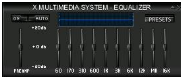
Abbildung 12-3. Xmms Equalizer
