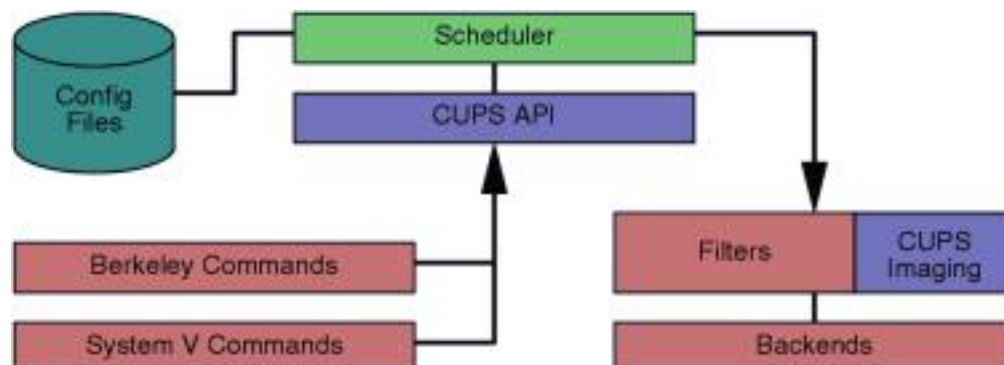
Abbildung 8-1. CUPS Diagramm
