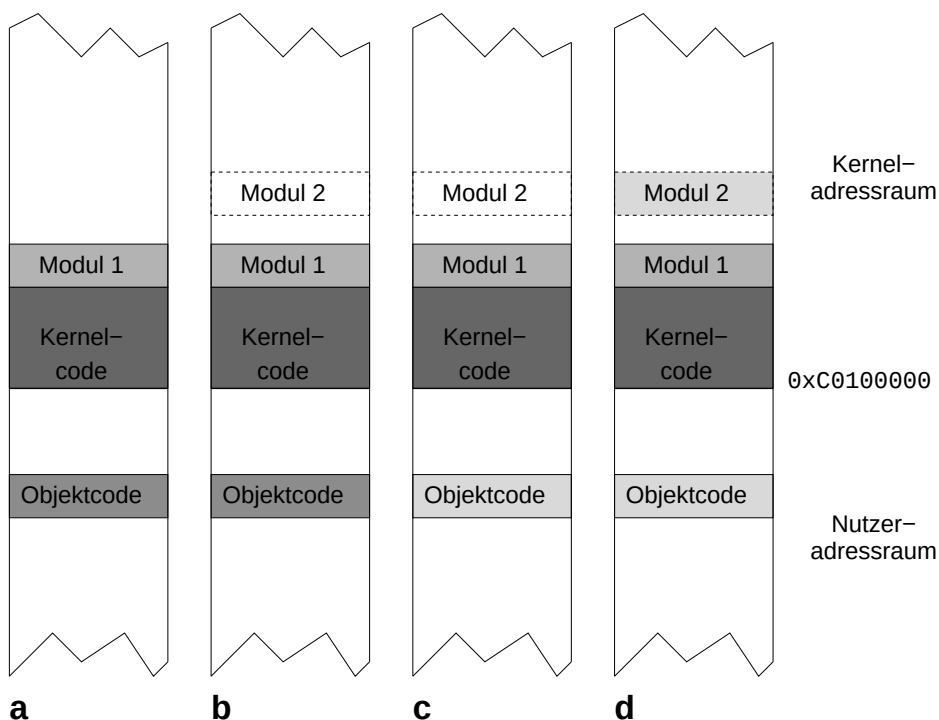
Abbildung 9.1: Der Adressraum beim Laden eines Moduls
