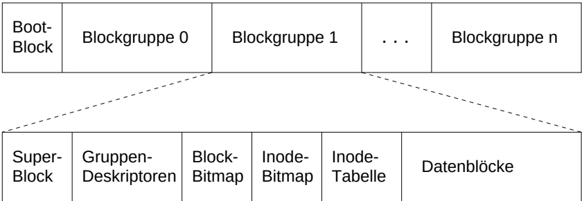
Abbildung 6.4: Der Aufbau des Ext2 -Dateisystems.
