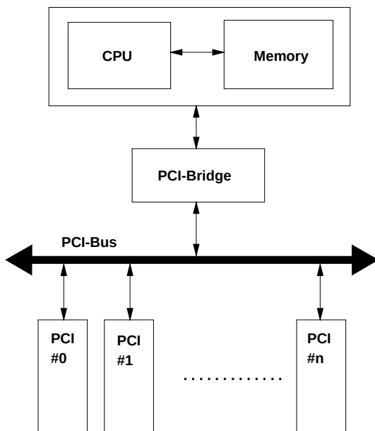
Abbildung 7.1: Schematischer Aufbau des PCI-Subsystems
