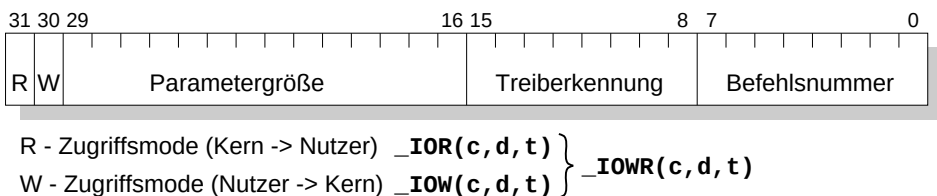
Abbildung 7.5: Kodierung der ioctl -Kommandos
