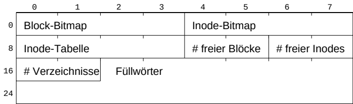
Abbildung 6.6: Die Blockgruppendesriptoren des Ext2-Dateisystems.
