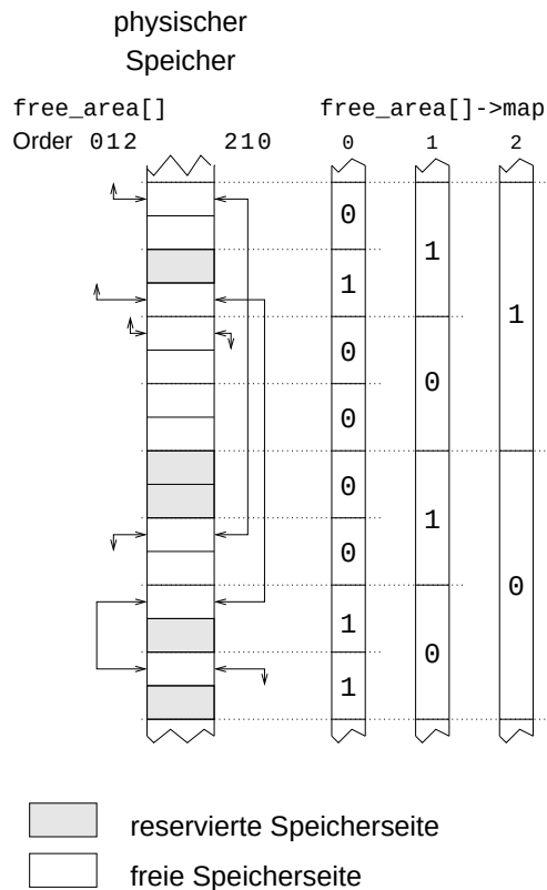
Abbildung 4.4: Beispiel der Belegung von free_area-Maps
