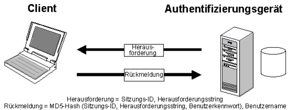
Abbildung 6: Der CHAP-Prozess
