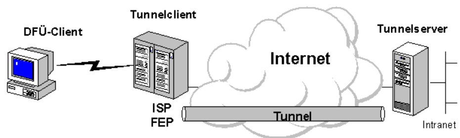
Abbildung 9: Erzwungener Tunnel
