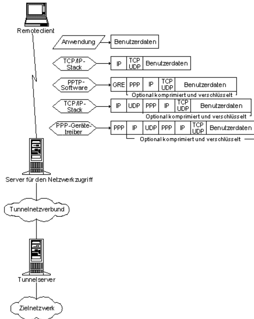
Abbildung 7. Aufbau eines PPTP Pakets
