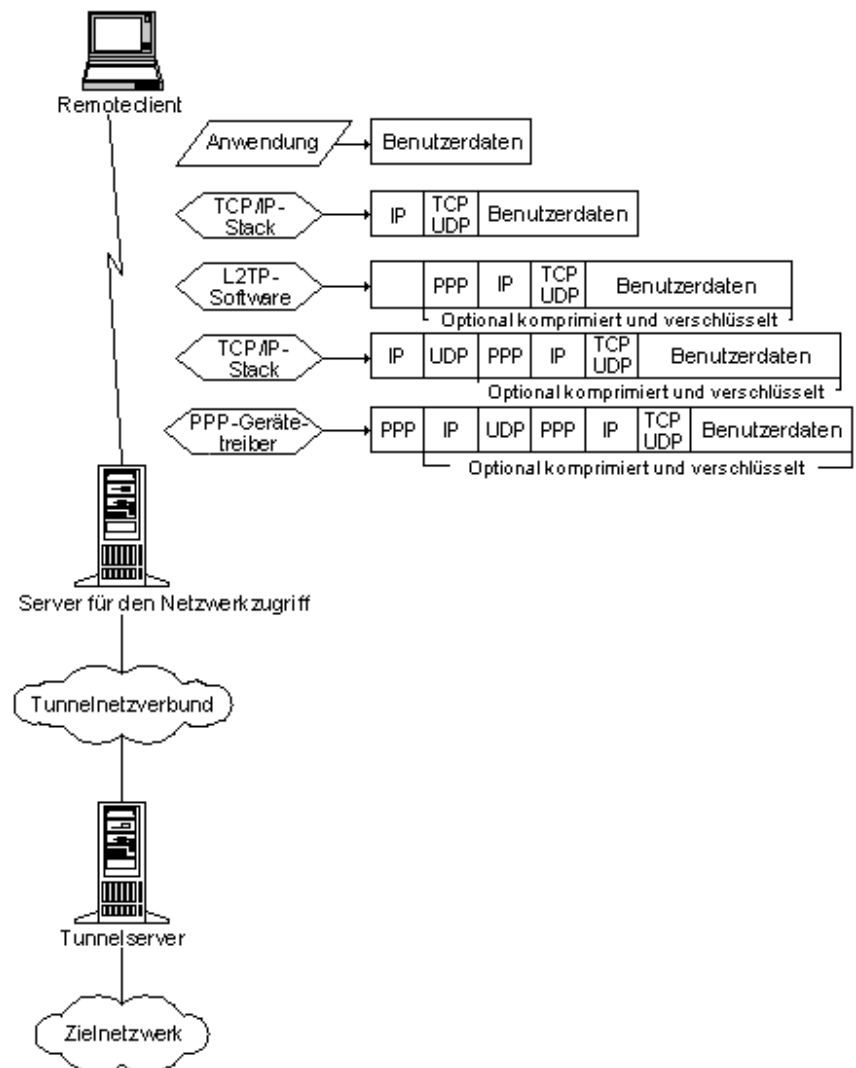
Abbildung 8. Aufbau eines L2TP-Pakets
