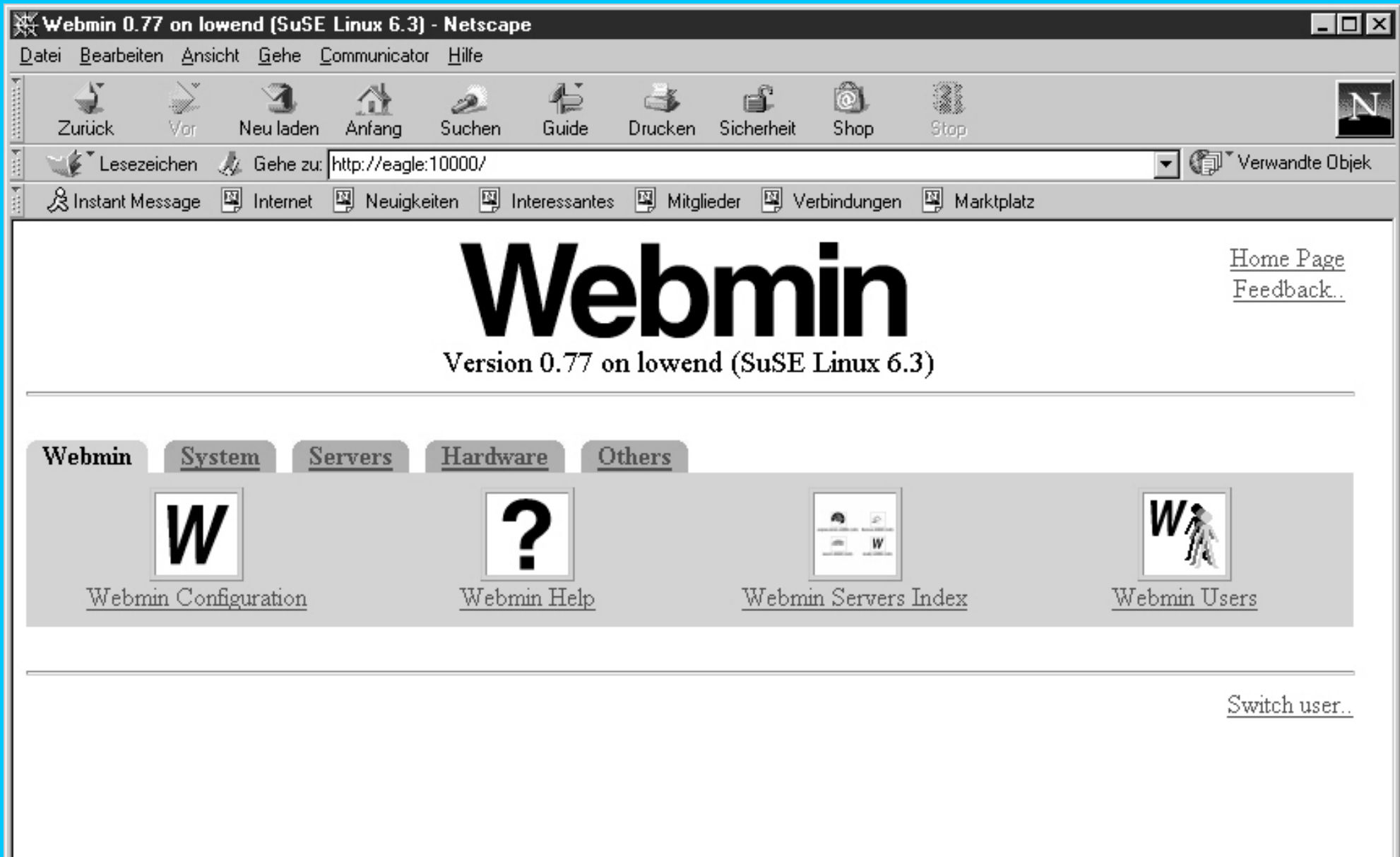
Abb. 9.12: Die Webmin-Homepage
