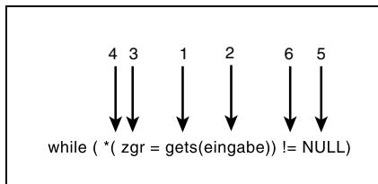
Abbildung 10.1: Die Komponenten der while -Anweisung, die auf leere Eingaben testet
