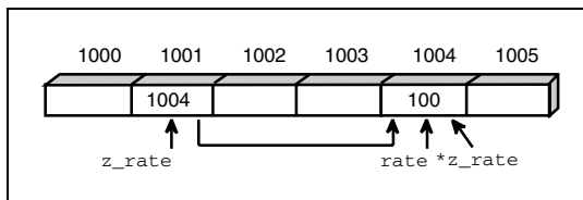
Abbildung 9.4: Der Indirektionsoperator vor Zeigern
