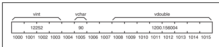
Abbildung 9.5: Verschiedene Typen der numme- rischen Variablen haben einen unter- schiedlichen Speicherbedarf
