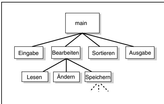
Abbildung 5.2: Ein strukturiertes Programm ist hierarchisch organisiert
