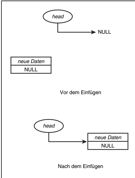
Abbildung 15.9: Einfügen eines neuen Elements in eine leere Liste
