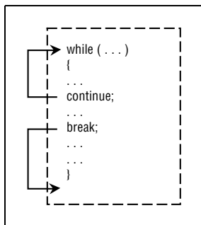
Abbildung 13.1: Der Ablauf der break - und continue -Anweisungen
