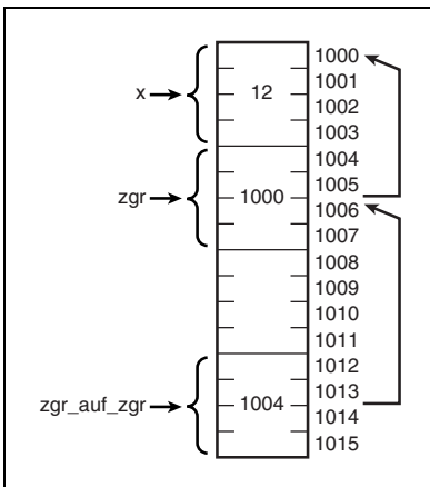
Abbildung 15.1: Ein Zeiger auf einen Zeiger
