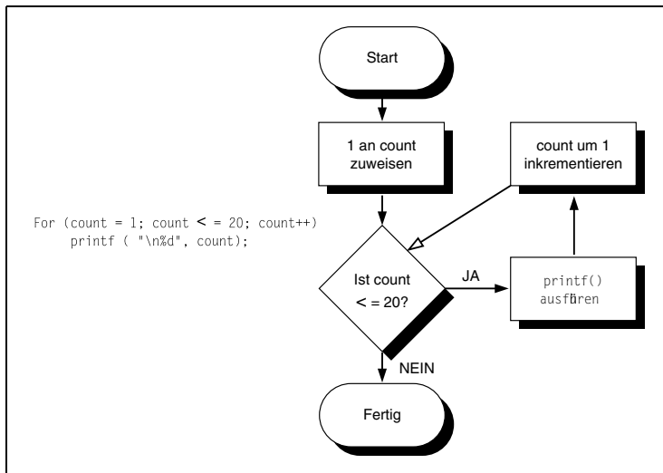
Abbildung 6.2: Funktionsweise der for-Schleife in Listing 6.1
