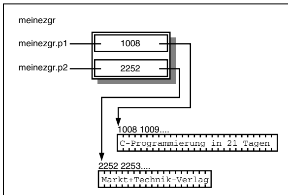
Abbildung 11.4: Eine Struktur mit Zeigern auf char
