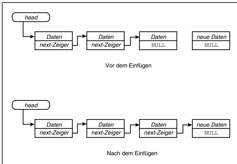
Abbildung 15.11: Einfügen eines neuen Elements am Ende einer verketteten Liste
