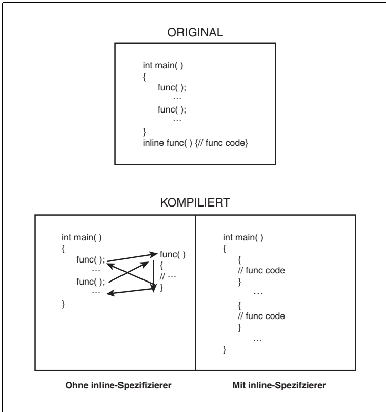
Abbildung 2.1: Inline-Funktionen und reguläre Funktionen
