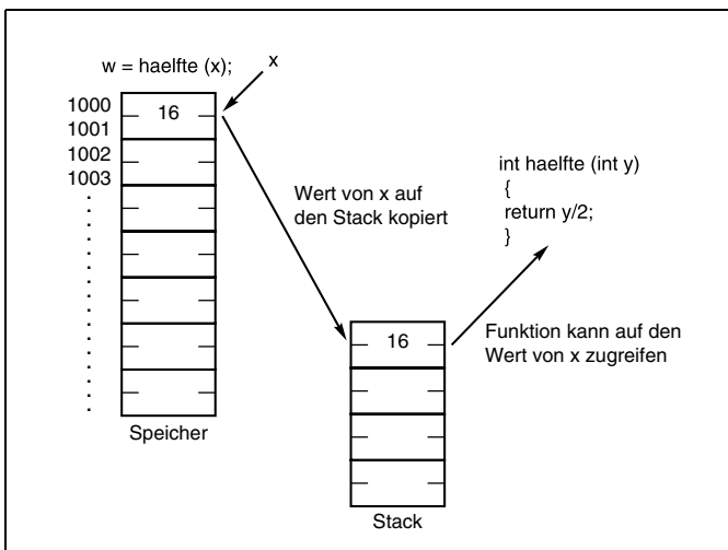
Abbildung 18.1: Ein Argument als Wert übergeben. Die Funktion kann den originalen Wert der Argumentvariablen nicht verändern
