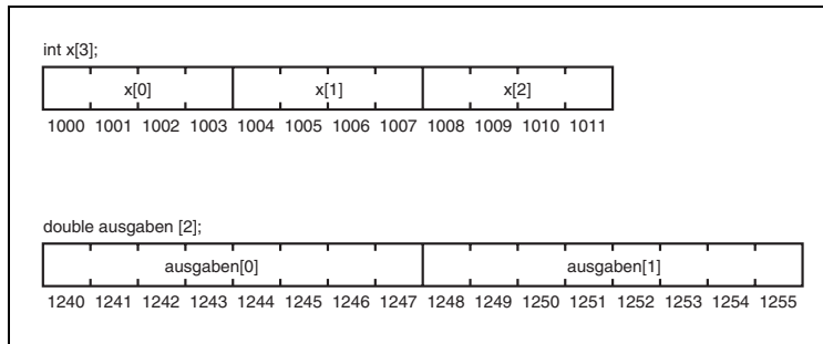
Abbildung 9.7: Arrays verschiedener Typen im Speicher
