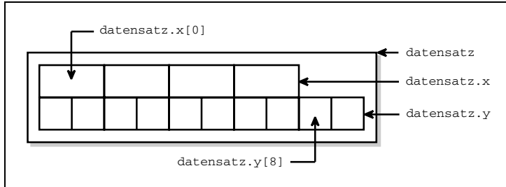
Abbildung 11.2: Der Aufbau einer Struktur, die Arrays als Elemente enthält
