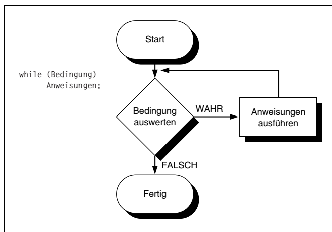
Abbildung 6.3: Ablauf der Programmausführung in einer while -Anweisung
