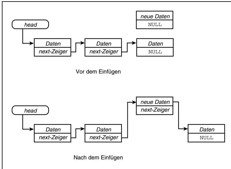
Abbildung 15.12: Einfügen eines neuen Elements in der Mitte einer Liste
