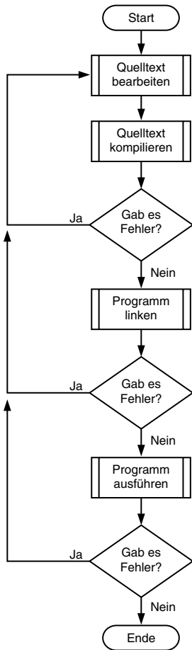
Abbildung 1.2: Die Schritte im Entwicklungszyklus eines C-Programms
