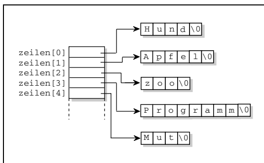
Abbildung 15.5: Vor dem Sortieren sind die Zeiger in der gleichen Reihenfolge im Array abgelegt, in der die Strings eingegeben wurden
