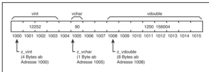
Abbildung 9.6: Der Compiler kennt die Größe der Variablen, auf die der Zeiger verweist
