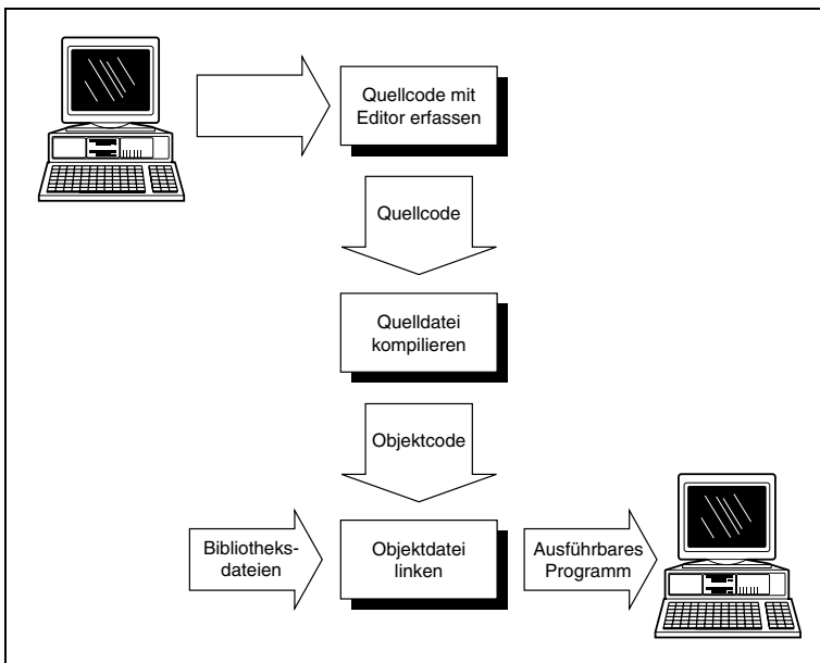
Abbildung 1.1: Den von Ihnen verfassten C- Quellcode konvertiert der Compiler in den Objektcode und der Linker produziert daraus die ausführbare Datei
