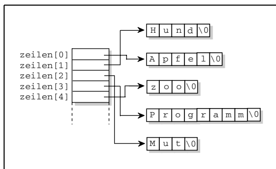
Abbildung 15.6: Nach dem Sortieren sind die Zeiger in alphabetischer Reihenfolge der Strings angeordnet
