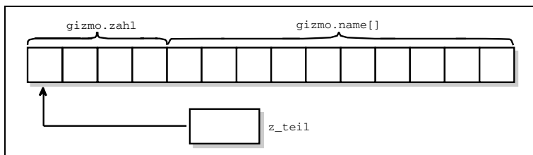
Abbildung 11.5: Ein Zeiger auf eine Struktur zeigt auf das erste Byte der Struktur
