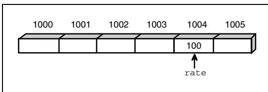
Abbildung 9.1: Eine Programmvariable ist an einer speziellen Speicheradresse abgelegt
