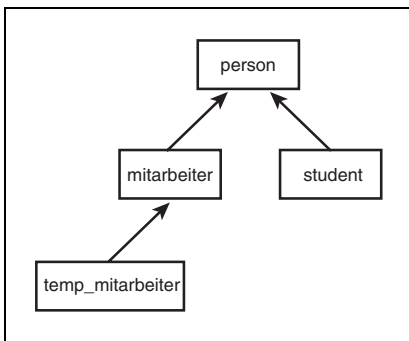
Abbildung 4.2: Eine Vererbungshierarchie
