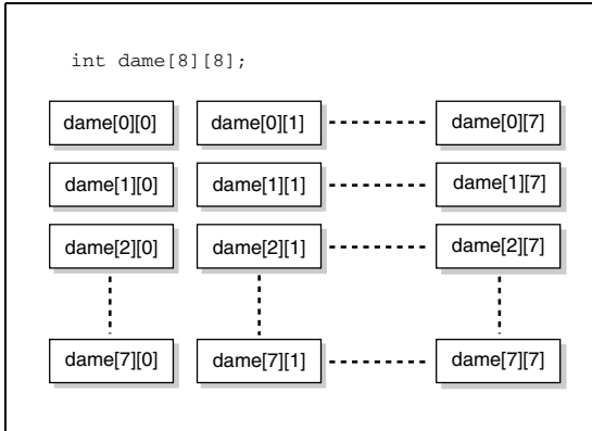
Abbildung 8.3: Ein zweidimensionales Array mit einer Reihen/Spalten-Struktur
