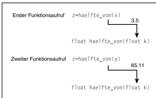
Abbildung 5.4: Bei jedem Funktionsaufruf werden die Argumente den Parametern der Funktion übergeben
