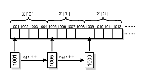
Abbildung 11.6: Mit jeder Inkrementierung rückt der Zeiger um ein Array-Element weiter
