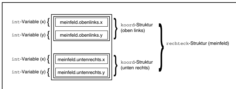
Abbildung 11.1: Die Beziehung zwischen einer Struktur, den Strukturen in die- ser Struktur und den Strukturele- menten
