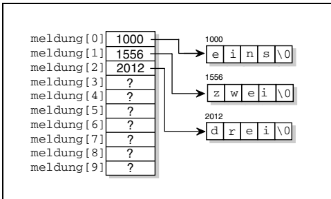
Abbildung 15.4: Ein Array von Zeigern auf char
