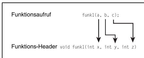
Abbildung 5.5: Mehrere Argumente werden den Funktionsparametern entsprechend ihrer Reihenfolge zugewiesen
