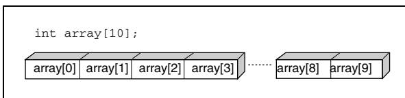
Abbildung 8.2: Array-Elemente werden hintereinander im Speicher abgelegt
