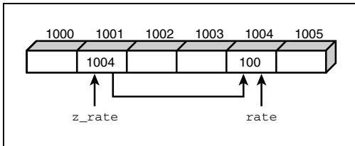
Abbildung 9.3: Die Variable z_rate enthält die Adresse der Variablen rate und ist deshalb ein Zeiger auf rate
