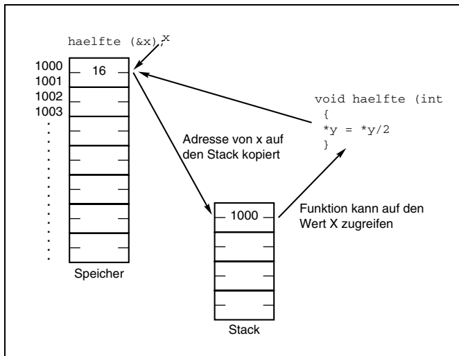
Abbildung 18.2: Die Übergabe als Referenz erlaubt einer Funktion, den originalen Wert der Argumentvariablen zu ändern
