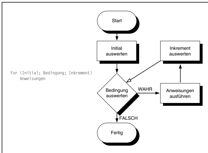
Abbildung 6.1: Schematische Darstellung einer for-Anweisung
