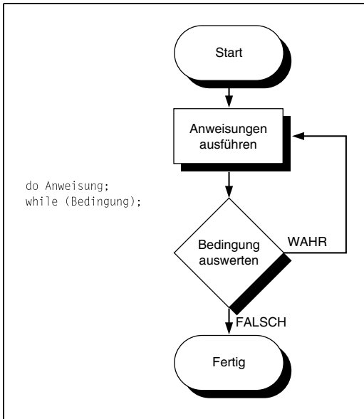
Abbildung 6.4: Die Abläufe in einer do...while-Schleife
