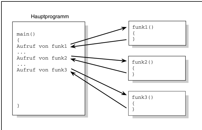
Abbildung 5.1: Wenn ein Programm eine Funktion aufruft, springt die Programmausführung in die Funktion und kehrt anschließend wieder zum aufrufenden Programm zurück
