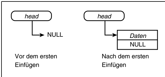
Abbildung 15.8: Der Kopfzeiger einer verketteten Liste
