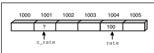
Abbildung 9.2: Der Compiler hat für die Variable z_rate Speicher reserviert
