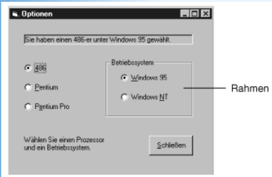
Abbildung 7.9: Wenn Sie eine Gruppe Optionsfelder in einem Rahmen anlegen, kann der Benutzer ein Optionsfeld im Rahmen und eines im Formular selektieren.
