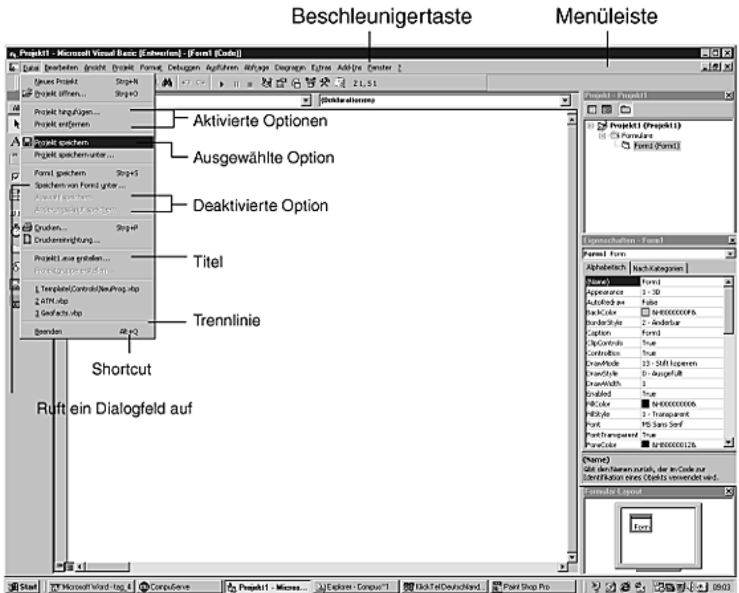
Abbildung 4.2: Visual Basic legt für Sie ein Standard-Windows-Menü und seine Optionen an.
