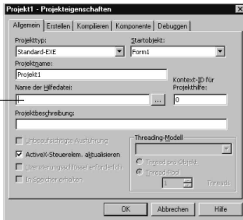
Abbildung 20.8: Hier verbinden Sie die Hilfedatei mit Ihrem Projekt.
