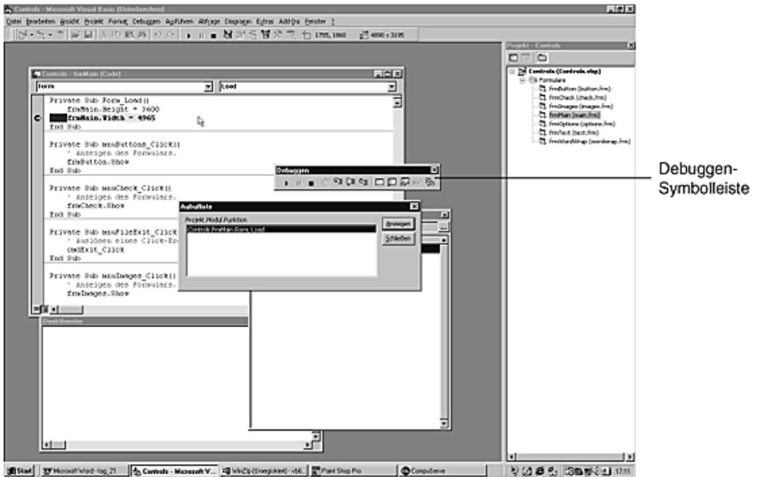
Abbildung 21.5: Im Dialogfeld Aufrufliste sehen Sie, welche Prozeduren in Ihrem Programm bisher ausgeführt wurden.
