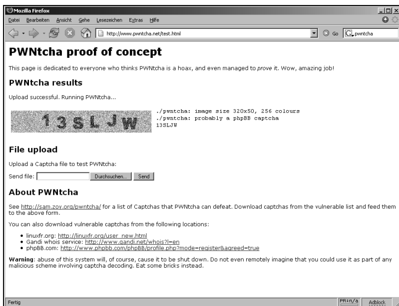
Abb. 6–1 CPTCHAs knacken mit PWntcha
