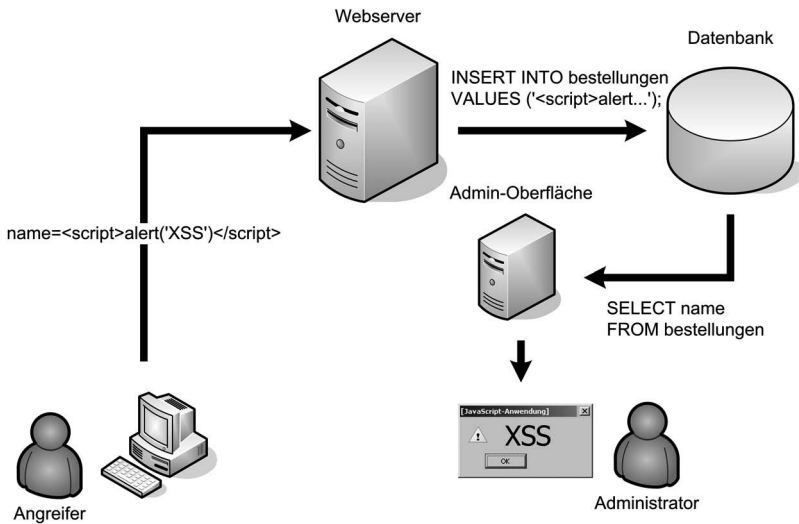
Abb. 4-1 XSS im LAN
