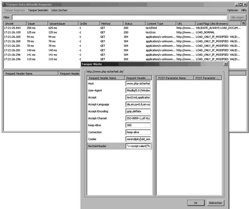
Abb. 3-1 Die Firefox-Extension »Tamper Data«
