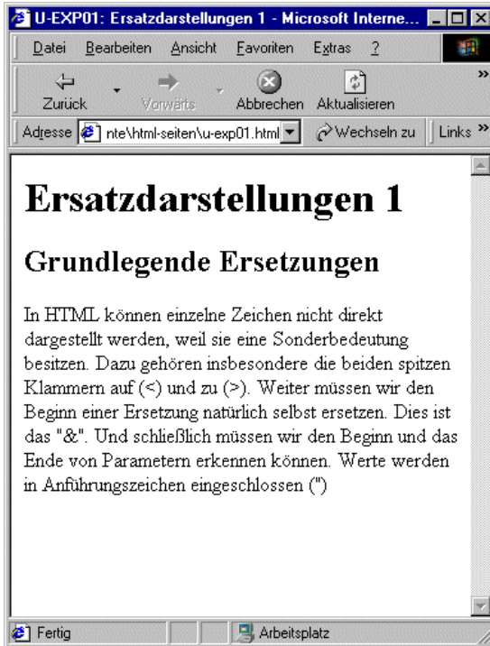
Abbildung 9.1: Grundlegende Ersetzungen
