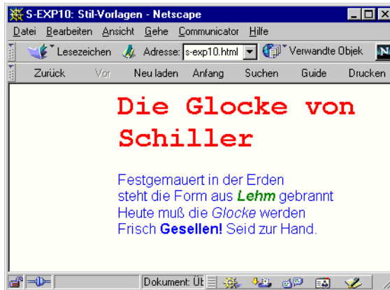
Abbildung 20.10: Direkt Stilanweisungen
