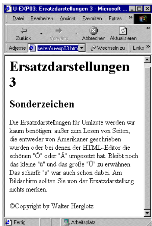
Abbildung 9.3: Numerische Ersatzdarstellung
