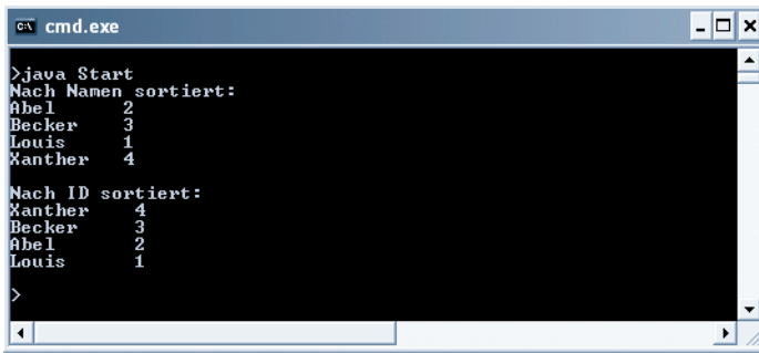
Abbildung 170: Sortieren mit verschiedenen Comparator-Objekten
