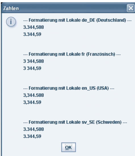
Abbildung 125: Zahlenformatierungen; die erste Zeile wurde jeweils mit einer getNumberInstance() -Instanz, die zweite Zeile mit einer DecimalFormat -Instanz formatiert.
