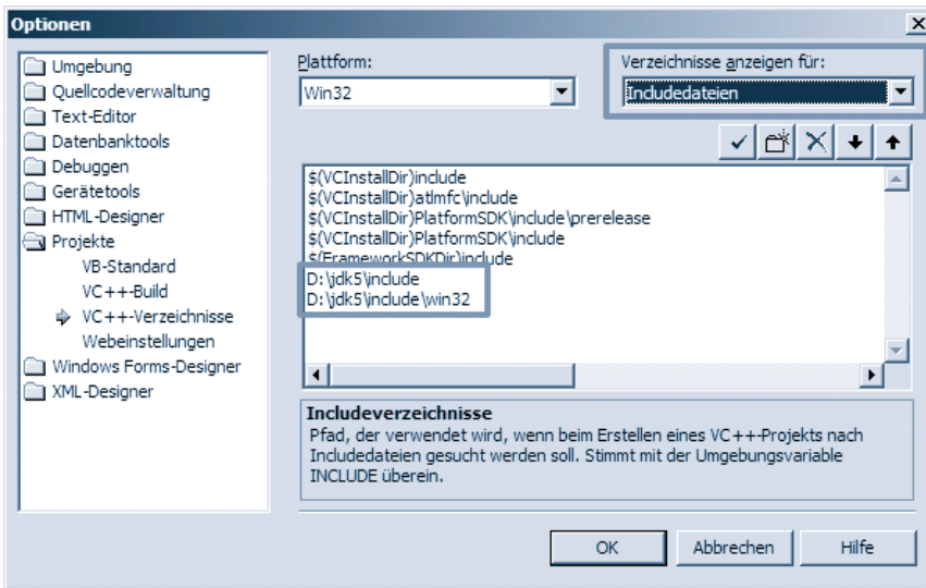
Abbildung 40: Hinzufügen der Java-Include-Verzeichnisse zum Projekt
