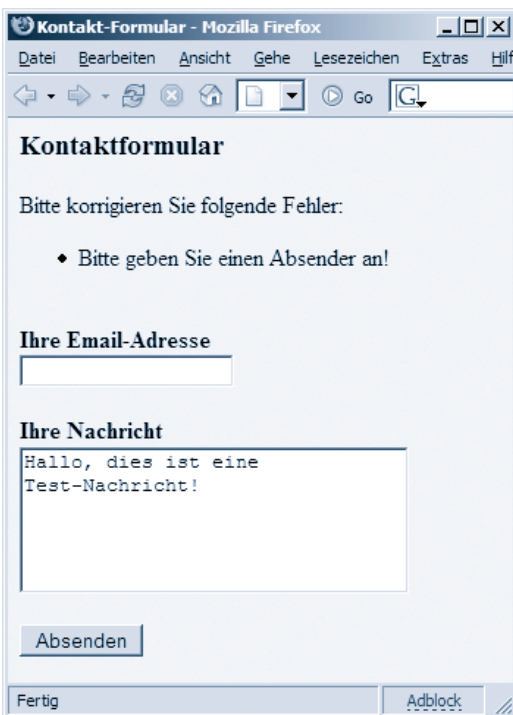
Abbildung 162: Der Absender fehlt.
