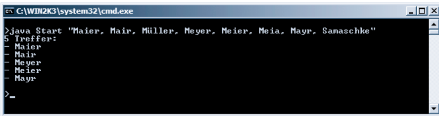
Abbildung 98: Ausgabe aller Treffer eines regulären Ausdrucks
