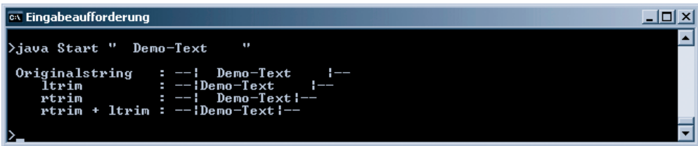
Abbildung 21: Effekt der Methoden ltrim() und rtrim()
