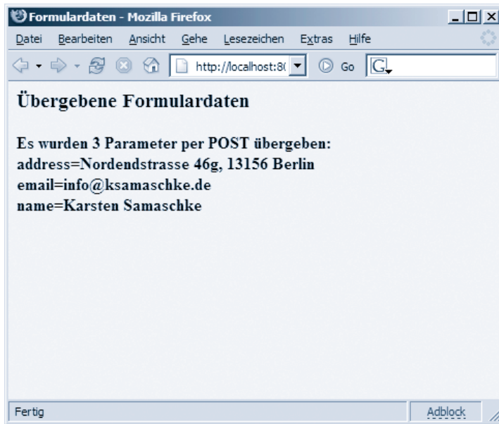
Abbildung 152: Ausgabe aller übermittelten Parameter
