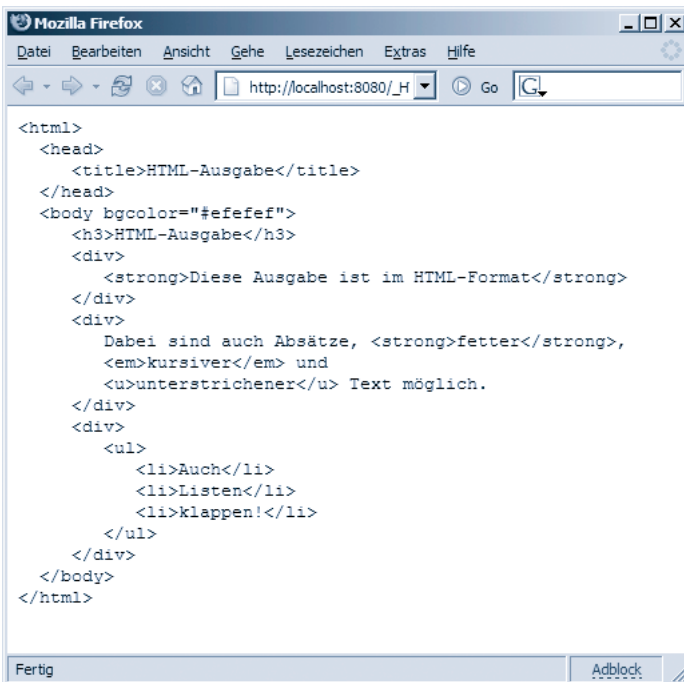
Abbildung 147: Rückgabe des Servlets in reiner Textdarstellung
