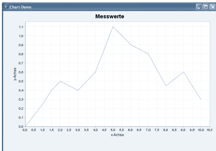
Abbildung 96: X-Y-Plot
