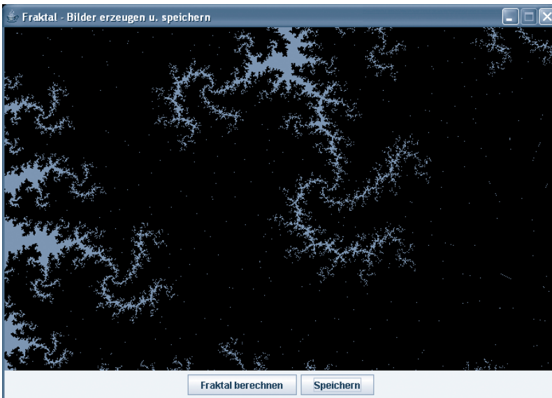
Abbildung 91: Julia-Menge
