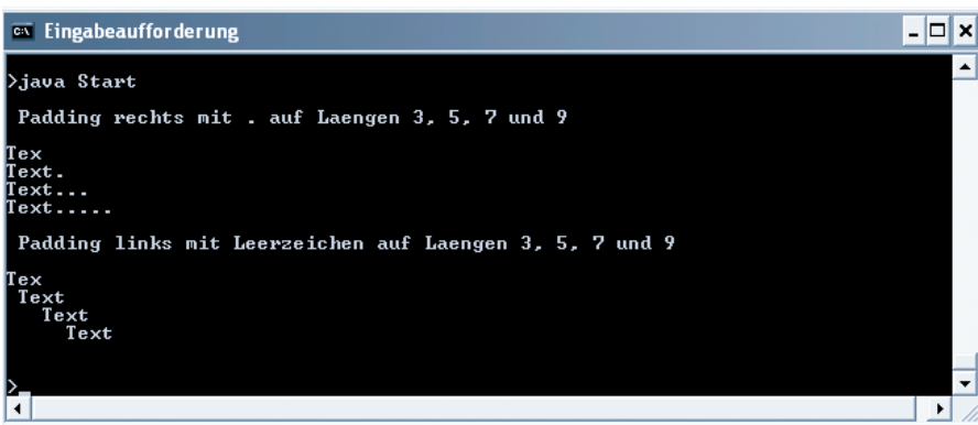
Abbildung 20: String-Padding
