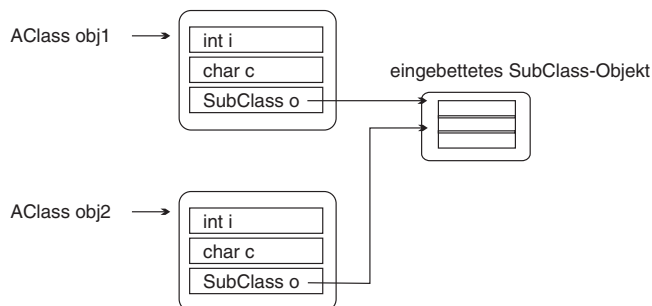
Abbildung 165: Flache Kopie
