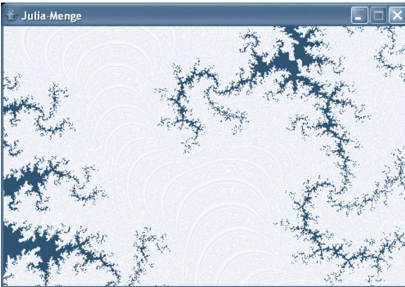
Abbildung 12: Julia-Menge
