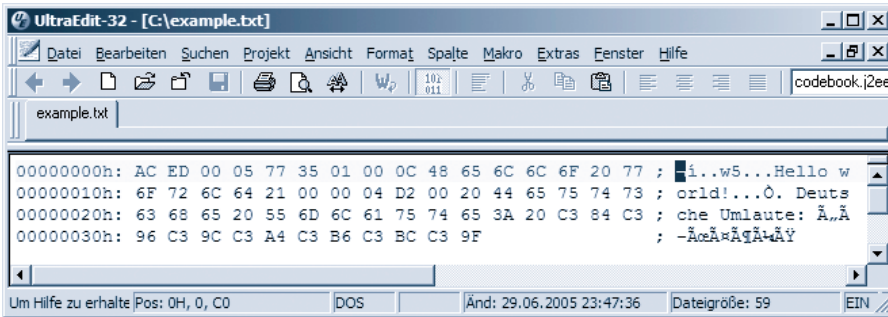
Abbildung 169: Anzeige der per ObjectOutputStream geschriebenen Daten
