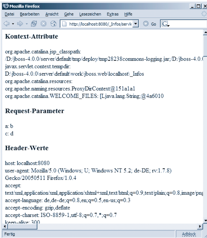
Abbildung 145: Ausgabe von Informationen aus dem Kontext eines Servlets
