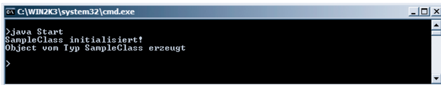
Abbildung 180: Ausgaben beim Erzeugen einer Klasseninstanz per Reflection
