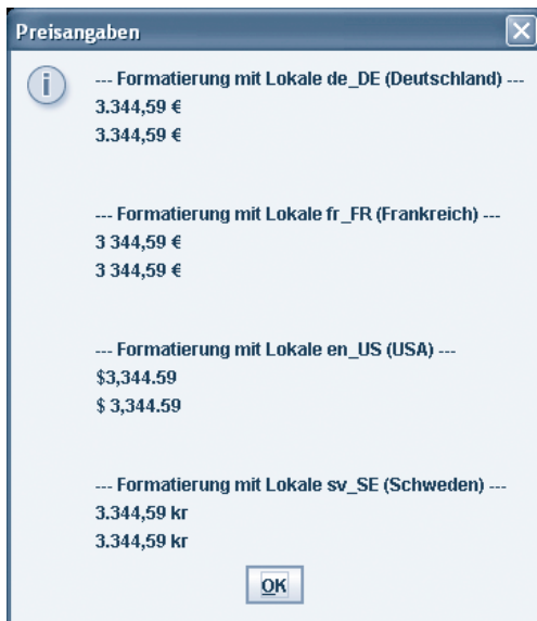
Abbildung 126: Formatierung von Währungsangaben; die erste Zeile wurde jeweils mit einer getCurrencyInstance() -Instanz, die zweite Zeile mit einer DecimalFormat -Instanz formatiert.
