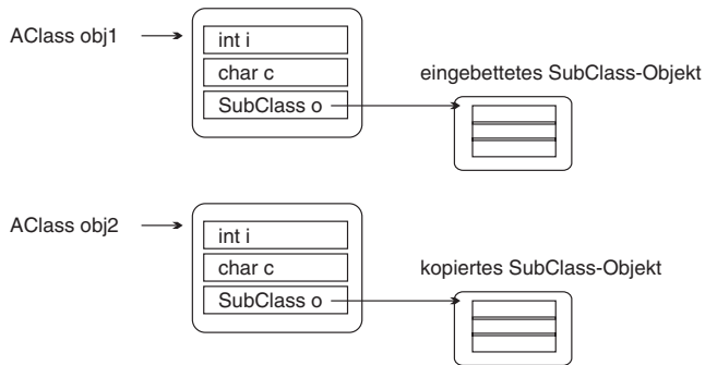
Abbildung 166: Tiefe Kopie
