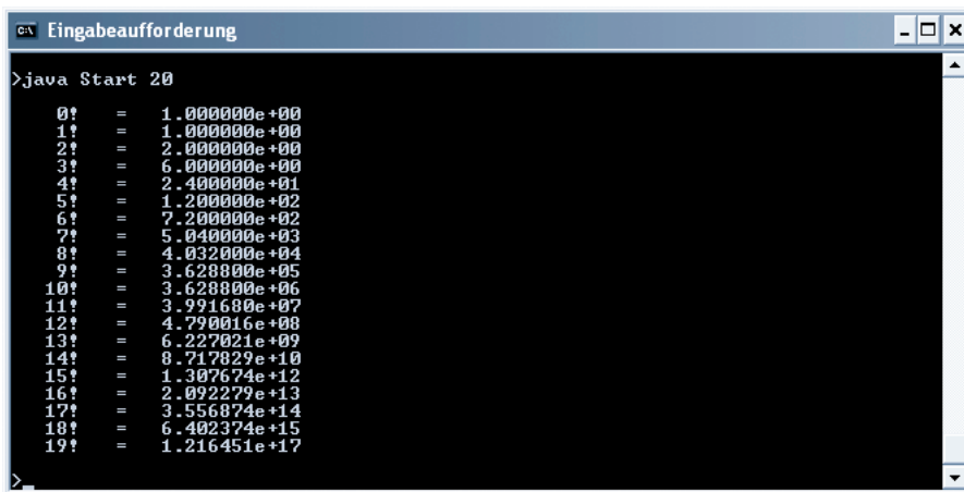
Abbildung 9: Fakultät
