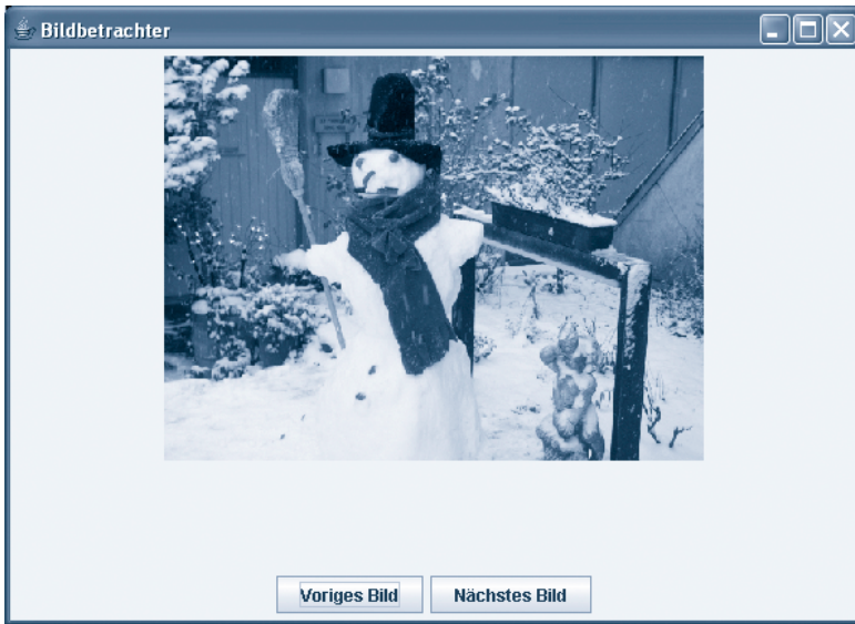
Abbildung 90: Diashow
