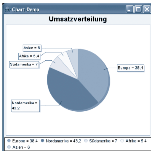
Abbildung 95: Tortendiagramm
