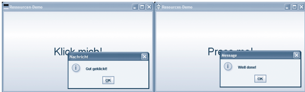
Abbildung 128: Das Programm zu diesem Rezept für die Lokalen de_DE und en_GB
