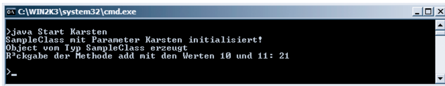
Abbildung 182: Die Methode add() wurde dynamisch eingebunden.
