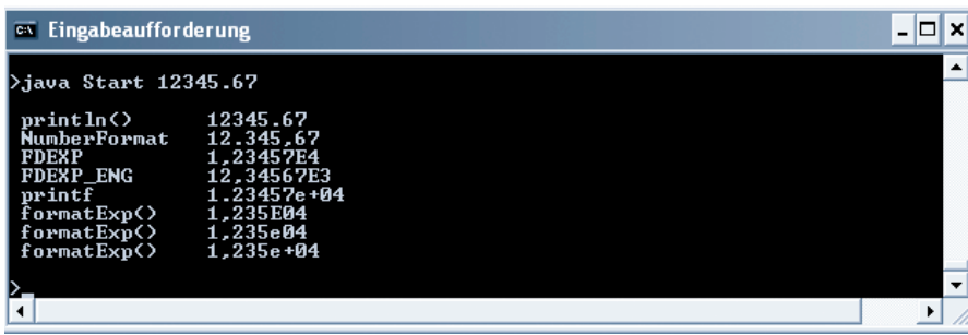
Abbildung 2: Formatierung von Dezimalzahlen
