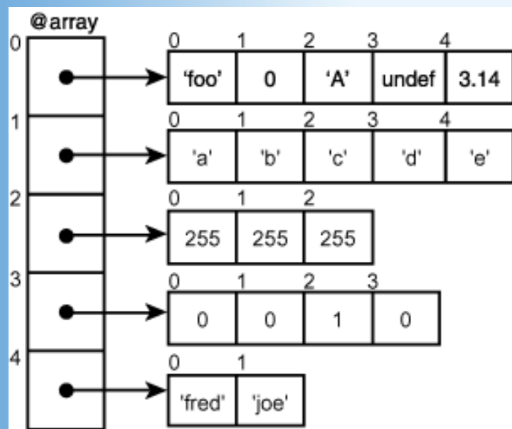
Abbildung 19.2: Ein Array von Arrays
