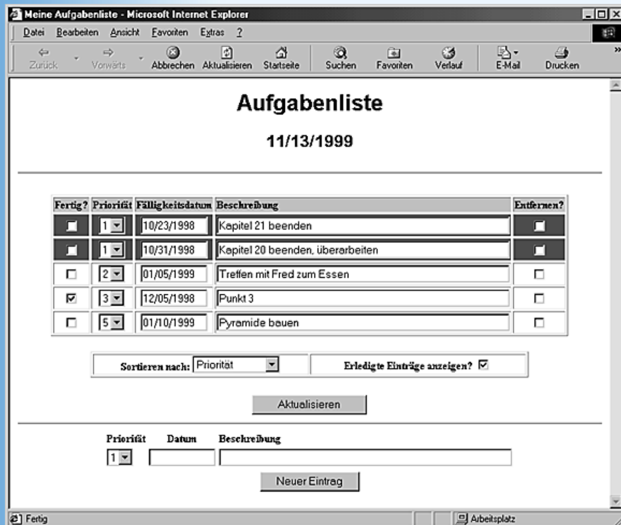
Abbildung 21.3: Die Web-Anwendung einer Aufgabenliste
