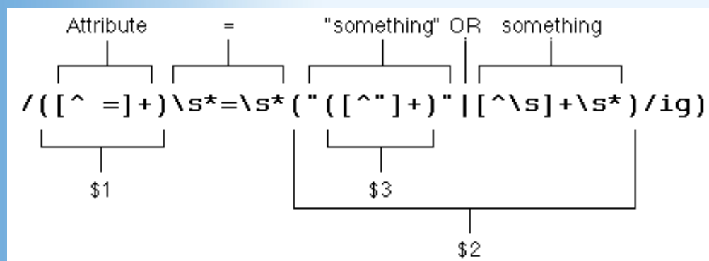
Abbildung 10.1: Die Teile des regulären Ausdrucks in img.pl
